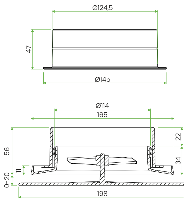
Anemostat z talerzykiem kwadratowym
