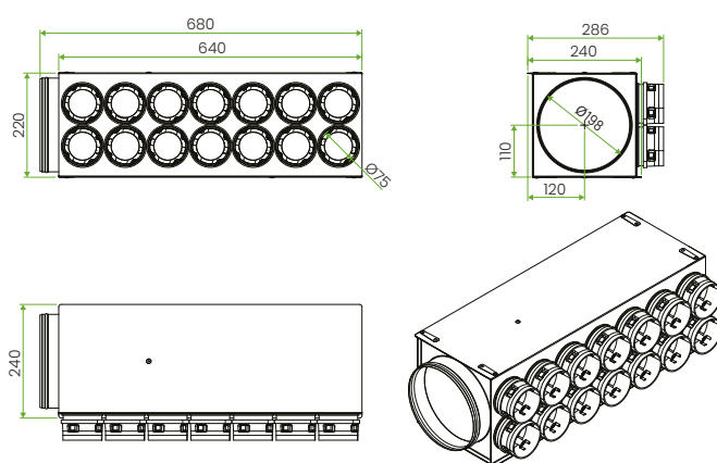
NCOS - rozdzielacz dwurzędowy kierunkowy - 14x75/198 mm
