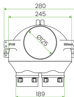
wersja podłogowa
