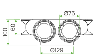
wersja sufitowa
