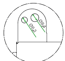
Uchwyt montażowy
