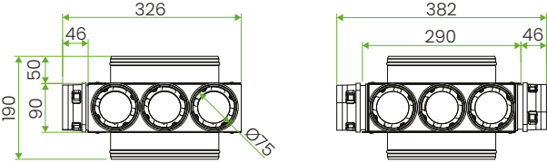
NCOX – rozdzielacz płaski góra/dół – 9x75/198 mm
