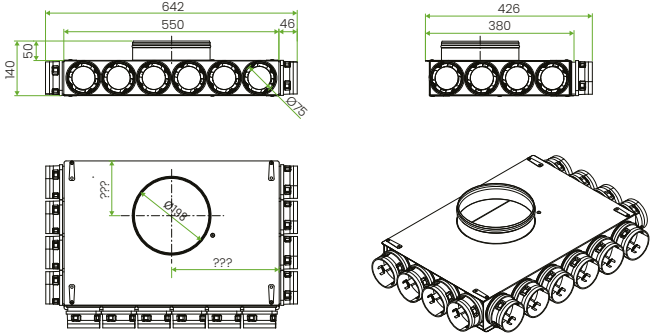
NCPE – rozdzielacz płaski – 14x75/198mm
