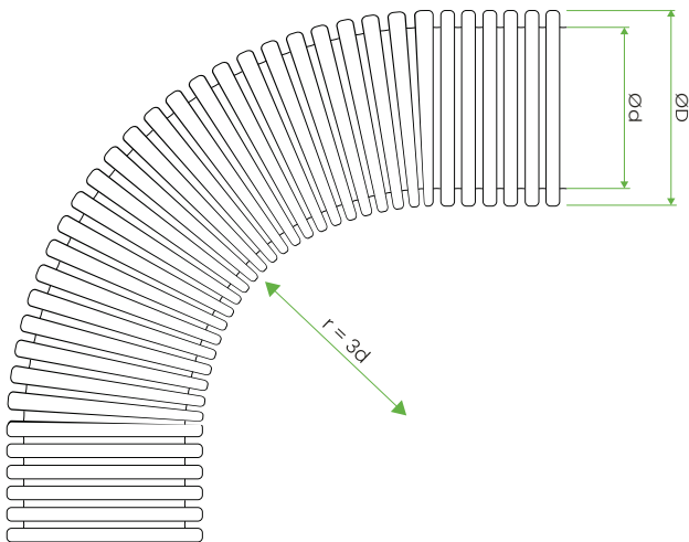
Promień zgięcia kanału okrągłego
