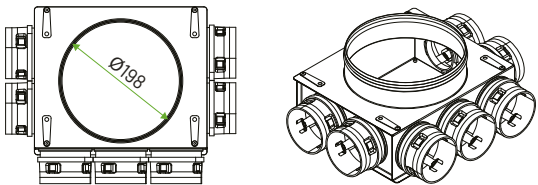
NCOW – rozdzielacz płaski – 9x75/198 mm
