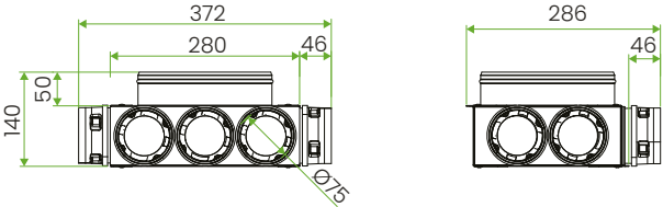
NCPC – rozdzielacz płaski – 7x75/198 mm
