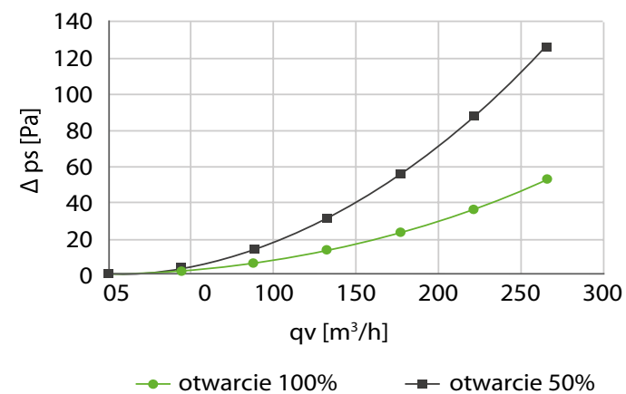
Wywiewna charakterystyka aerodynamiczna anemostatów PEFLEX PREMIUM Ø125 mm
