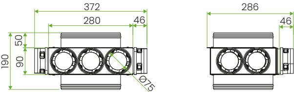
NCPD – rozdzielacz płaski góra/dół – 7x75/198mm
