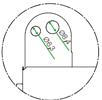
Uchwyt montażowy
