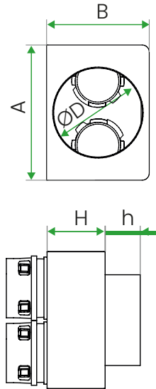
Uchwyt montażowy
